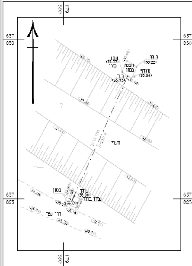
קנה מידה 1 : 250
